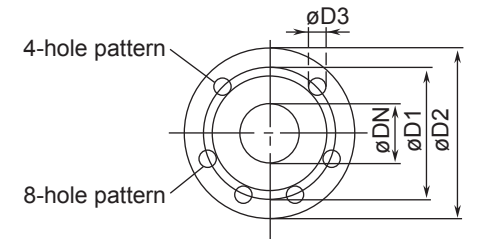
Flange dimensions EN 1092-2
