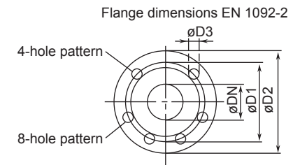
Flange dimensions in acc.with DIN EN 1092-2
